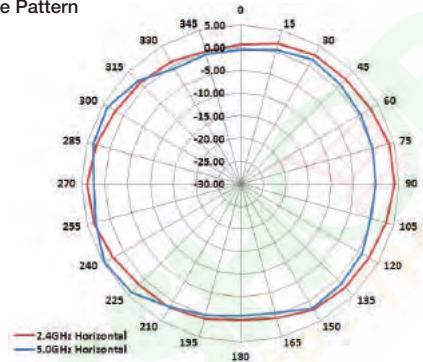
H-Plane Pattern
