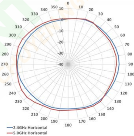
H-Plane Pattern
