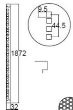
Thanh tiêu chuẩn
