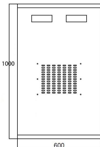
Mặt nóc tủ
